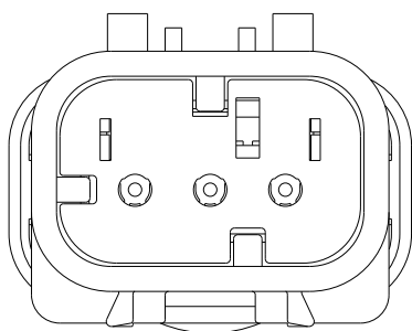
776535-4 SCALE 2:1 KEY D
