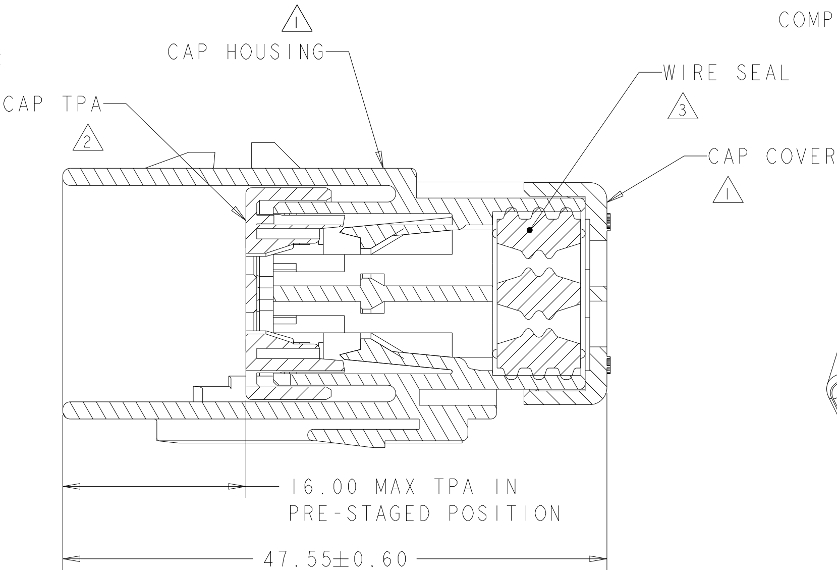
SECTION A-A
